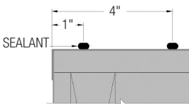
FIG. 8: OUT-SWING PATIO DOOR SILL
