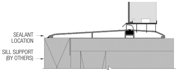
FIG. 16: HANDICAP DOOR SILL
